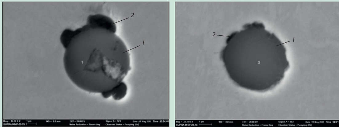
Рис. 4. Многофазные включения, обнаруженные в пробах металла, отобранных в процессе непрерывной разливки: 1 — основа — алюминаты кальция ( \text{CaO-Al}_2\text{O}_3 ); 2 — оксиды системы \text{FeO-Al}_2\text{O}_3
